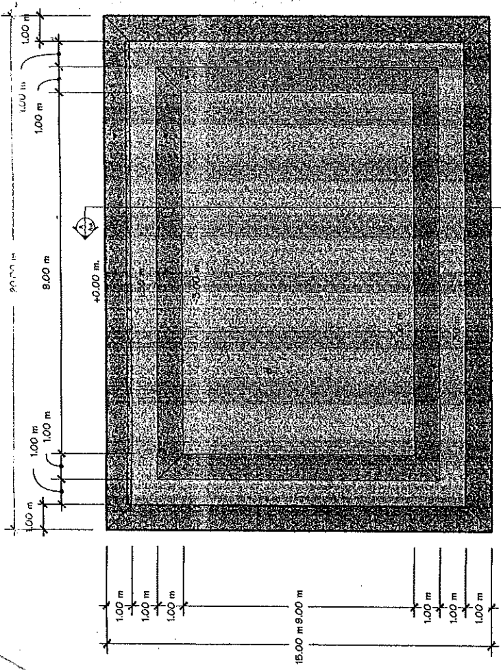
แปลนหน้าดินและตำแหน่งขุดหน้า NO:SCALE
